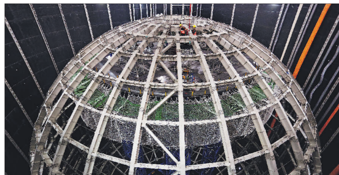
6月23日,江门中微子实验(JUNO)地下700米的实验大厅内,工程人员顺利完成试验装置主结构球形网壳的拼接。该装置计划于明年建成运行,将使我国成为国际中微子研究的中心之一。 黄继明 摄
