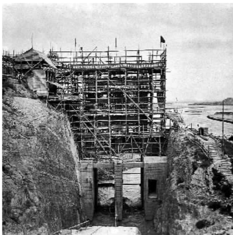
1953年,官厅水库进水塔进行第四期工程施工作业。(工人日报 侯印封 摄)
